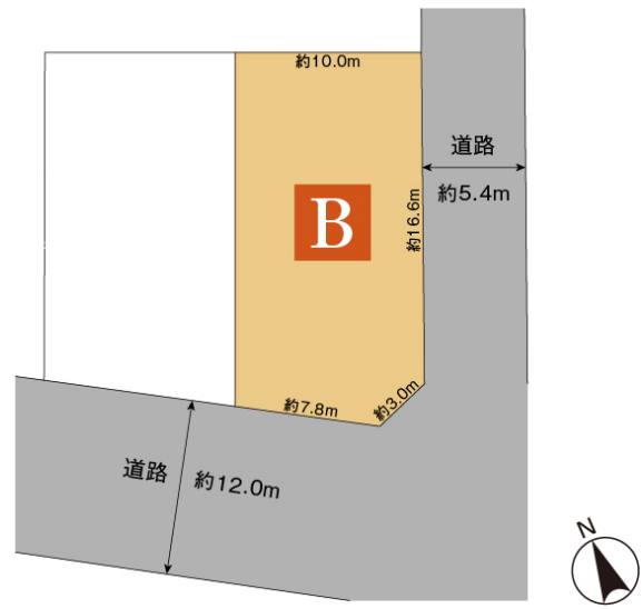
■ 区画図
